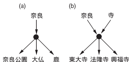
図2 連想構造
