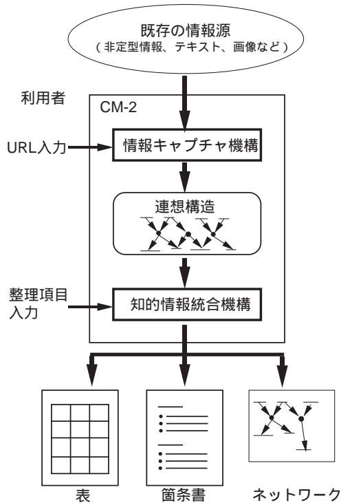
図3 Overview of CM-2 Fig. 3 CM-2 の概要
