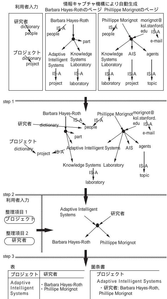
図6 知的情報統合機構のアルゴリズム動作例 Fig. 6 Intelligent Information Integration Facility
